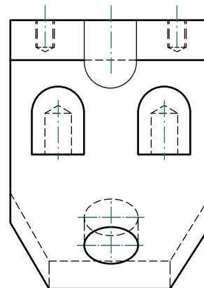
END ELEVATION
